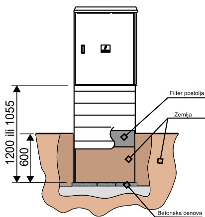
Način postavljanja uzemnog postolja
