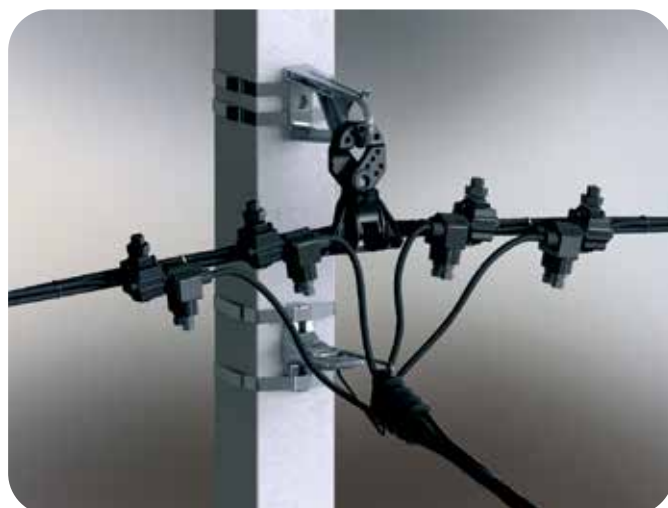
Noseće prihvatanje pomoću ES 1500 sa ocepom pomoću PC 4-150, FA 2, CA 1500 i PA 25
