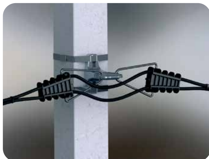
Zatezno prihvaćanje pomoću CA 1500 i PA 25
